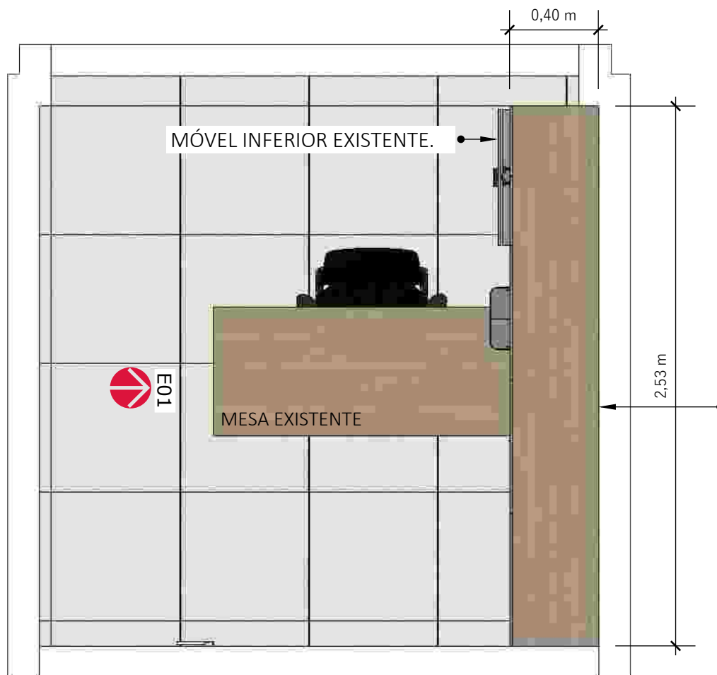
PLANTA BAIXA - SALA FRANCIS ESCALA _____ 1:25
