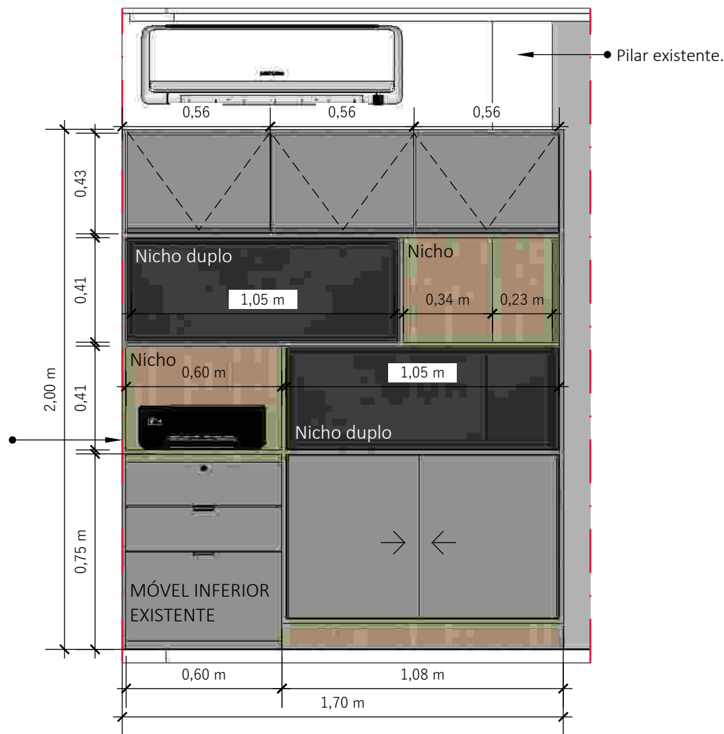
ELEVÇÃO 01 - ESTANTE ESCALA _____ 1:20
